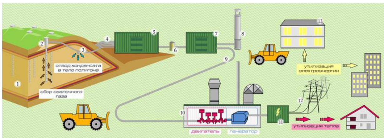
Рисунок 1. Структура полигона для сбора ТБО, обезвреживания и утилизации свалочного газа. Условные обозначения: 1. тело полигона; 2. газовая скважина; 3. Конденсатоотводчик; 4. газосборный трубопровод; 5. газосборная станция; 6. сборник конденсата; 7. компрессорная станция; 8. факельная установка; 9. газовый трубопровод; 10. когенерационная установка; 11. трансформаторная подстанция; 12. ЛЭП; 13. административное здание
