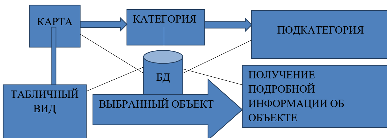
Рисунок 1. Схема распространения запросов (указаны линиями) и потоков данных (указаны стрелками) от базы данных к модулям приложения
