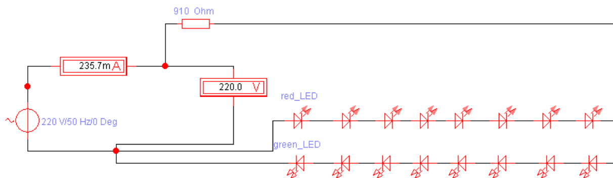
Рисунок 1. Схема включения светодиодного модуля в сеть с напряжением 220 В переменного тока промышленной частоты 50 Гц
